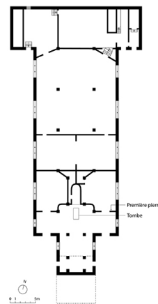
Plan de l'étage de soubassement, extrait cadastral de la Direction Générale des Finances Publiques (DGFIP) 2022, échelle 1/500e.
