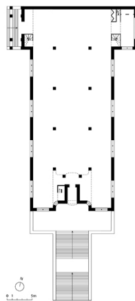
Plan du rez-de-chaussée, extrait cadastral de la Direction Générale des Finances Publiques (DGFIP) 2022, échelle 1/500e.
