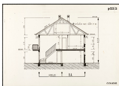
Projet de construction d'une maison d'habitation Camélia [recto et verso du plan], s.d. [1981]. Phot. Sonia Dourlot, Autr. Selam IVR43_20187000001NUC4A
