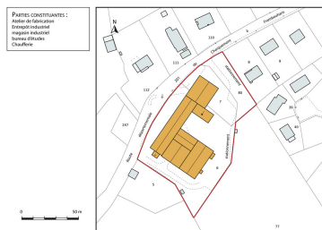
Plan-masse et de situation. Extrait du plan cadastral, 2013, section AM. Dess. Mathias Papigny
