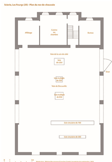
Plan du rez-de-chaussée, mise au net d'un relevé, 1/100, par E. Parrod, 1912. Dess. Aline Thomas IVR43_20212500157NUDA
