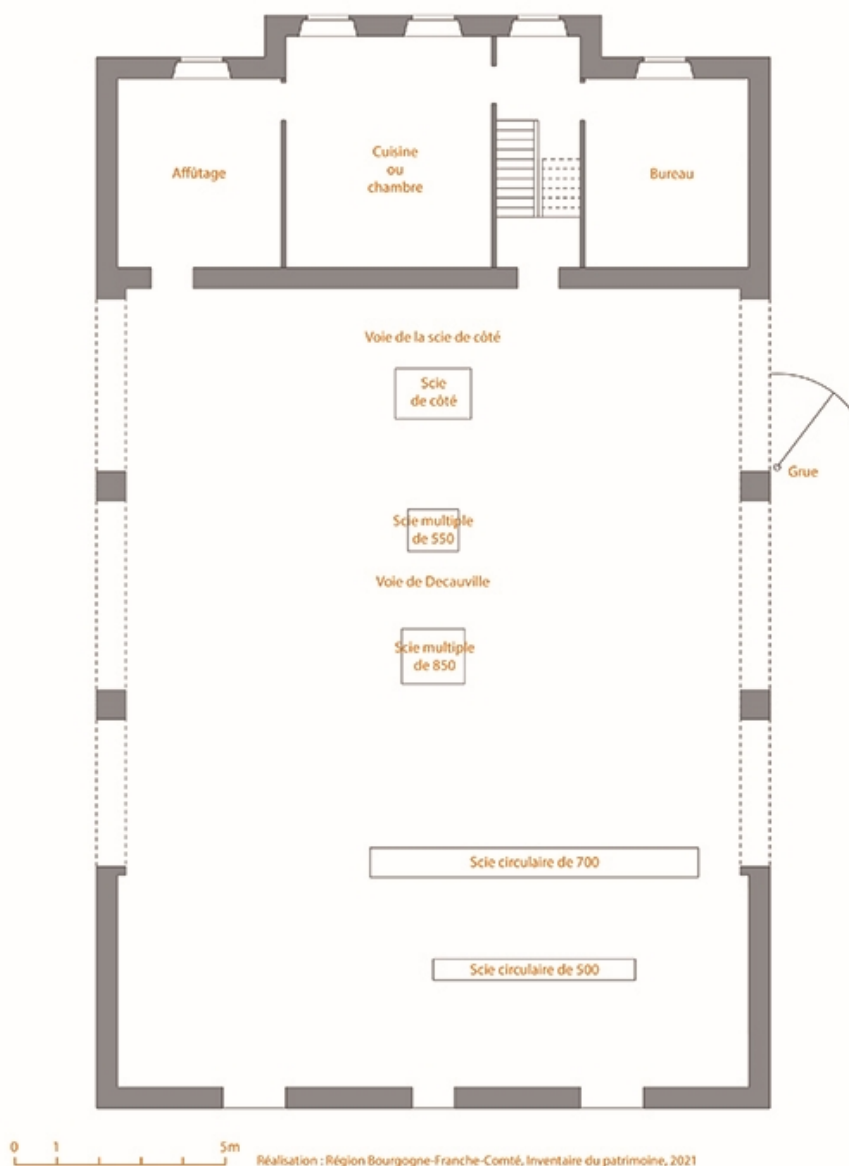
Scierie, Les Fourgs (25) - Plan du rez-de-chaussée
