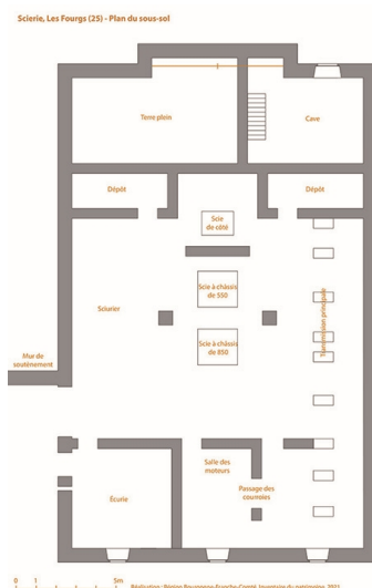
Plan du sous-sol, mise au net d'un relevé, 1/100, par E. Parrod, 1912. Dess. Aline Thomas IVR43_20212500156NUDA
