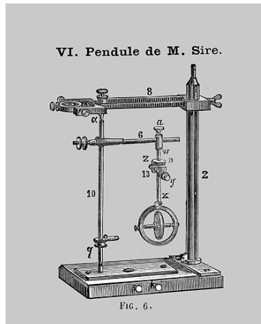
[Montage du stréphoscope :] VI - Pendule de M. Sire, 1883. Phot. Yves Sancey IVR43_20052500010X
