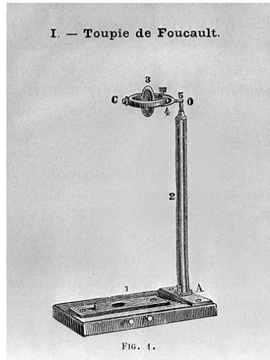
[Montage du stréphoscope :] I - Toupie de Foucault, 1883. Phot. Yves Sancey IVR43_20052500005X
