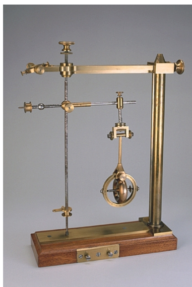
Montage : tourniquet alternatif à tension de M. Gruey. Phot. Jérôme Mongreville IVR43_20032500985XA
