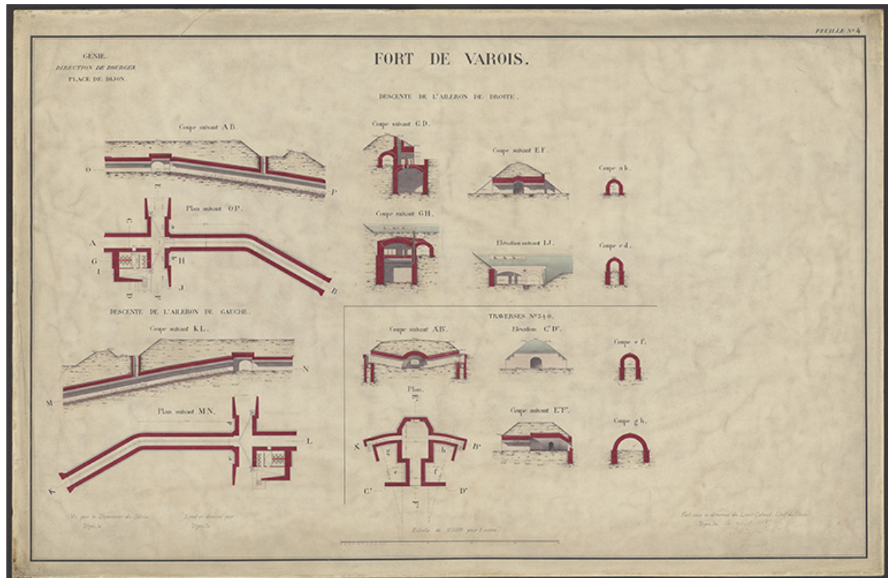
Fort de Varois. Descente de l'aileron de droite. 1885.
