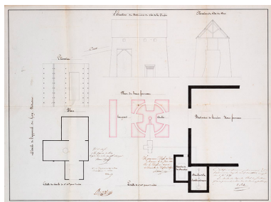
[Plans et élévations du haut fourneau de Clerval], 1842. Phot. Jérôme Mongreville IVR43_20152500590NUC4A
