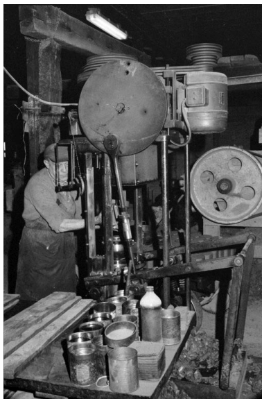
Mouleuse à pots de fleur CROCHON (5). Phot. Laurent Poupard IVR43_19883900354Z
