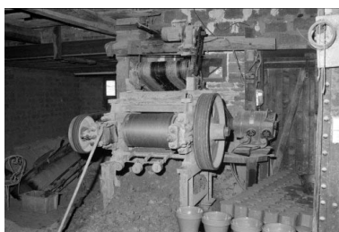
Broyeur UNICERAM (5). A droite, pâtons au sortir de la boudineuse et avant moulage. Phot. Laurent Poupard IVR43_19883900352Z
