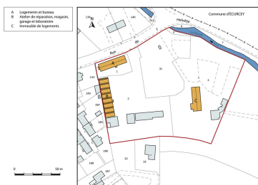
Plan-masse et de situation. Extrait du plan cadastral numérisé, section AN, échelle 1:1000. Dess. Mathias Papigny IVR43_20142500578NUDA
