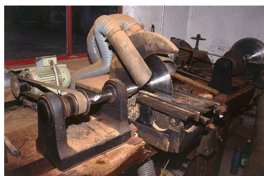
Vue d'ensemble de la scie de gauche, servant au calibrage (dressage des côtés). Phot. Jérôme Mongreville IVR43_20003901046ZA
