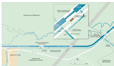
Plan schématique du réseau hydraulique des biefs 13 et 14 du versant Saône. Dess. Alain Morelière IVR26_20132100093NUDA
