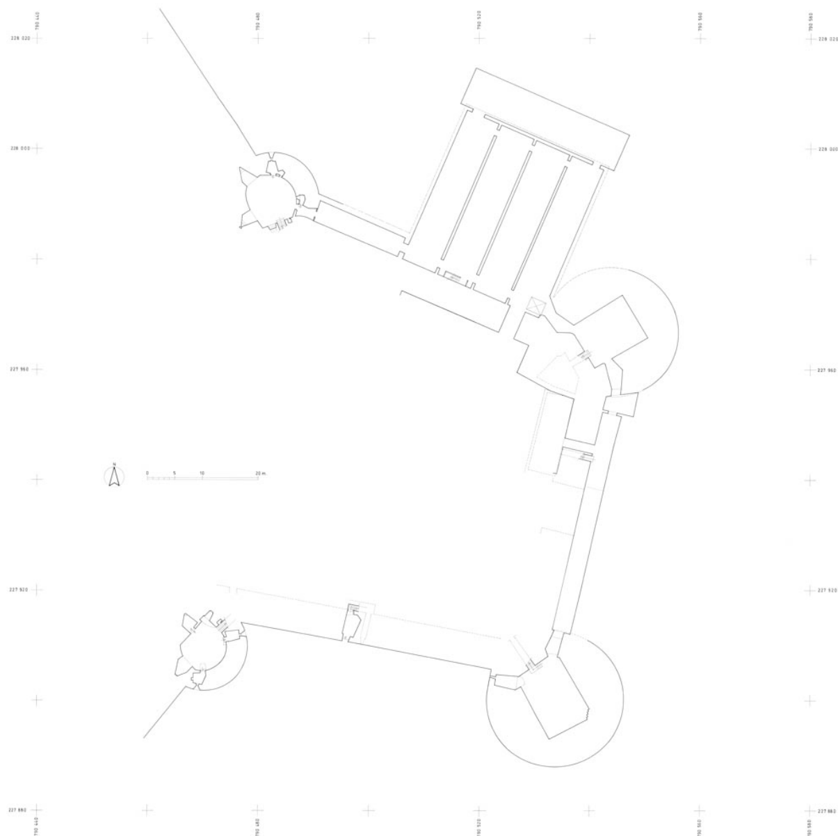
Plan du niveau supérieur.
