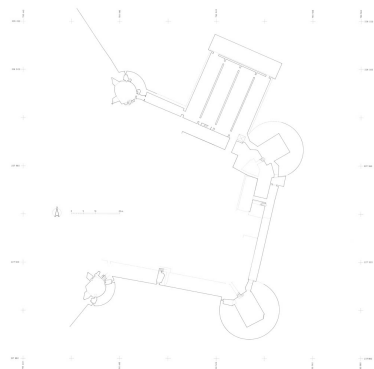
Plan du niveau supérieur.
