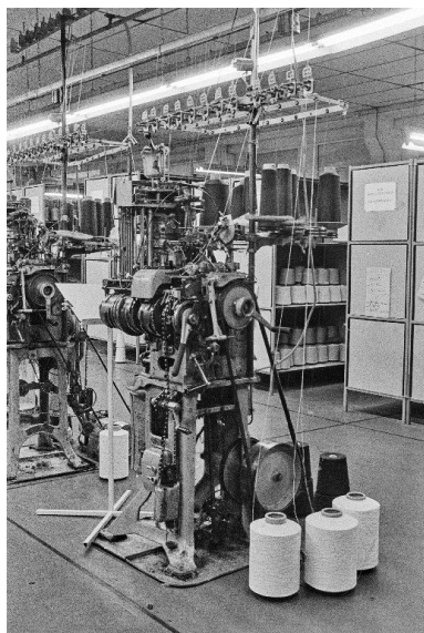
Machine à tricoter des chaussettes dite " Komet ", de type BC : vue d'ensemble. Phot. Frédéric Pillet IVR26_19997100254Z
