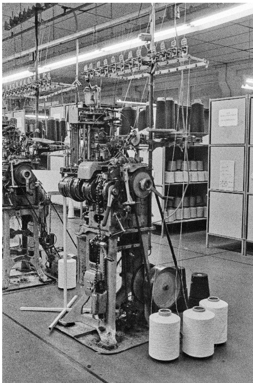
Machine à tricoter des chaussettes dite " Komet ", de type BC : vue d'ensemble.
