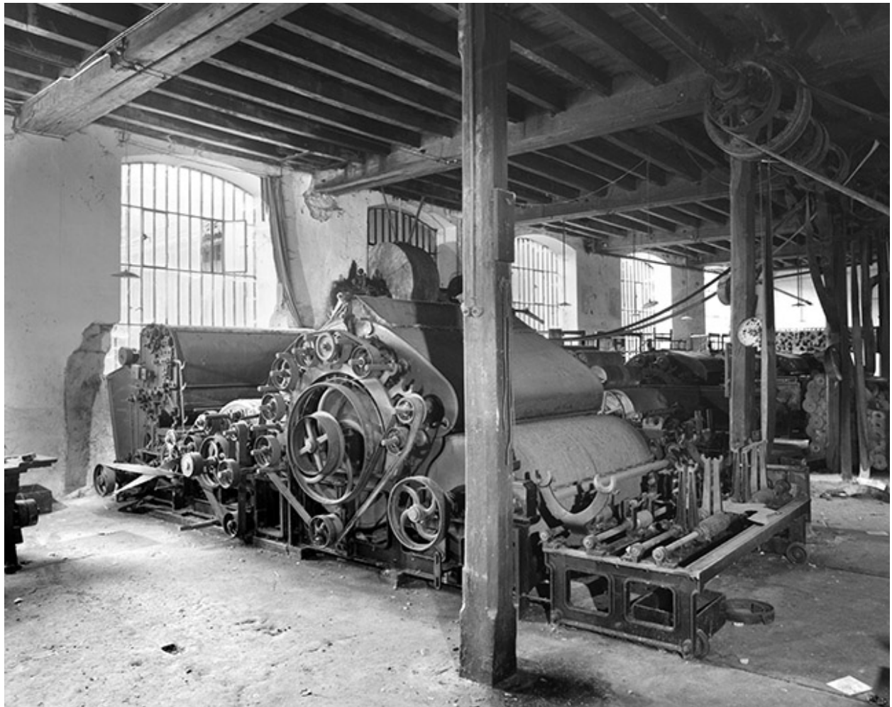
Vue d'ensemble : face arrière vue de trois quarts gauche.
