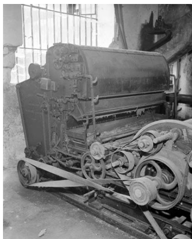
Chargeur peseur.
