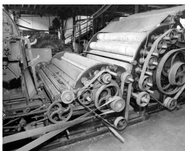
Cylindre briseur et avant-train.
