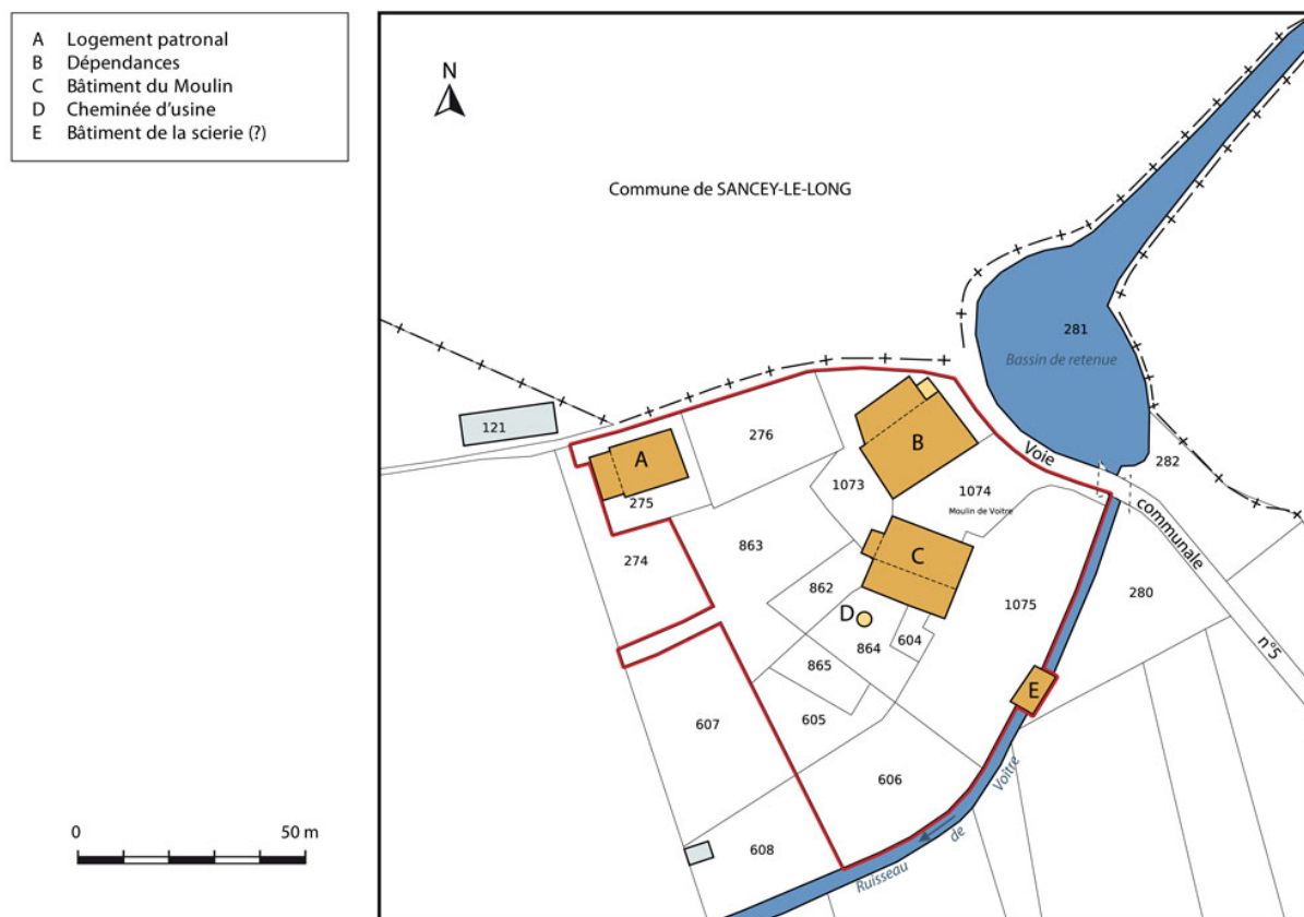
Plan-masse et de situation. Extrait du plan cadastral, 2015, section A.
