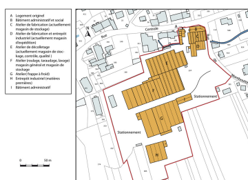
Plan-masse et de situation. Dess. Mathias Papigny IVR43_20132502565NUDA
