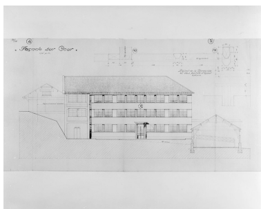
[Projet d'agrandissement de l'usine] Façade sur cour. Phot. Jérôme Mongreville, Phot. Lucien Fraenkel IVR43_19993900515V
