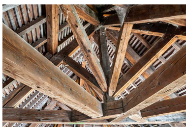
Charpente. Détail de l'enrayure sud. Phot. Jérôme Mongreville
