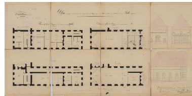
Plan présentant les innovations à exécuter dans les Appartemens de l'Hôtel de ville pour l'établissement d'une Salle d'assemblée. 6 mai 1828. Phot. Pierre-Marie Barbe-Richaud, Autr. Simon Tridon IVR26_20212100334NUC4A
