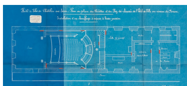
Hôtel de Ville de Châtillon-sur-Seine. Vue en plan du théâtre et du Rez-de-chaussée de l'Hôtel-de-Ville au niveau du Perron. Installation
