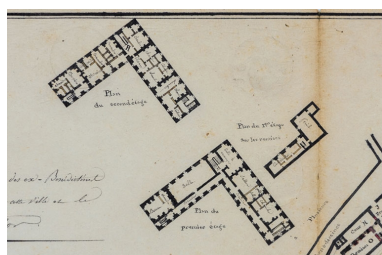
Plan des bâtiments des ex-Bénédictines de Châtillon-sur-Seine [...] Détail : 1er et 2e étages. S.d. [1821 ?].
