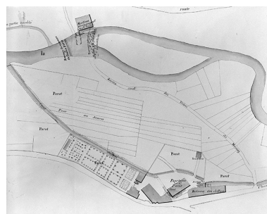
Plan des lieux. Révision du règlement d'eau de l'usine Parrot. Phot. Jérôme Mongreville IVR43_19963901789V
