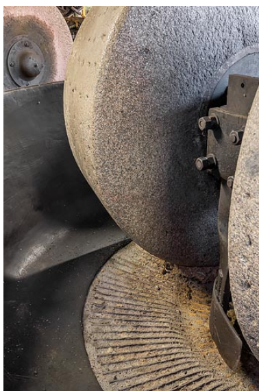
Défibreuse : détail des meules. Phot. Pierre-Marie Barbe-Richaud IVR43_20203900102NUC4A
