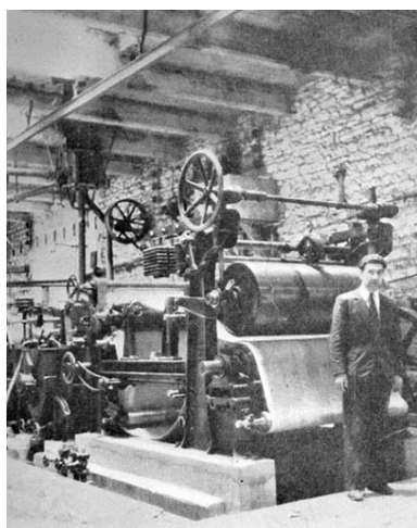
Machine enrouleuse. Phot. Jérôme Mongreville IVR43_19973900003X
