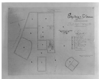
Plan pour demander l'autorisation de placer une machine à vapeur de 12 chevaux. Phot. Jérôme Mongreville, Phot. Charpy IVR43_19963901796V
