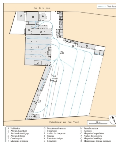
Plan-masse de l'usine en 1913.
