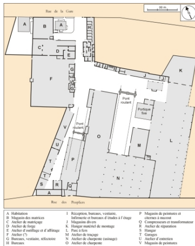
Plan-masse de l'usine en 1964. D'après un plan conservé dans les archives privées de l'entreprise, daté mai 1964, mis au net par A. Céréza. Dess. André Céréza IVR43_20057000167NUDA
