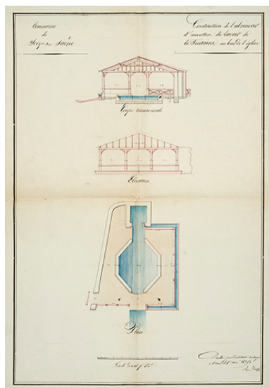
Construction de l'abreuvoir et couverture du lavoir de la fontaine au bas de l'église. 1835. Repro. Jérôme Mongreville, Autr. Charles Vincent Théodore Le Beuffe IVR43_2019700002NUC4A
