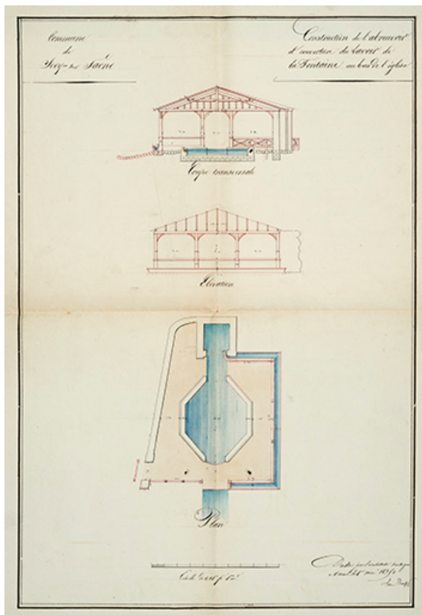
Construction de l'abreuvoir et couverture du lavoir de la fontaine au bas de l'église. 1835.
