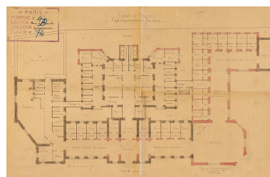
Projet de Naudet (1890). Repro. Pierre-Marie Barbe-Richaud, Autr. Charles Thomas Désiré Naudet IVR26_20205800295NUC4A
