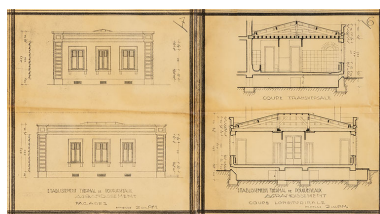
Projet de Massé et Riniéri (1934), coupes et élévations extérieures du pavillon à construire.
