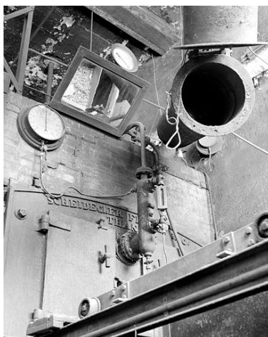
Détail de la partie haute de la chaudière de 1927 (cadrage vertical). Tuyau articulé de chargement de la trémie à droite ; rail et chariot de la trémie en bas. Phot. Yves Sancey IVR43_19999000235X
