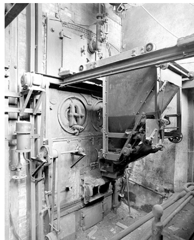
Détail de la porte de la chaudière de 1927, avec sa trémie à charbon. Phot. Yves Sancey IVR43_19999000234X
