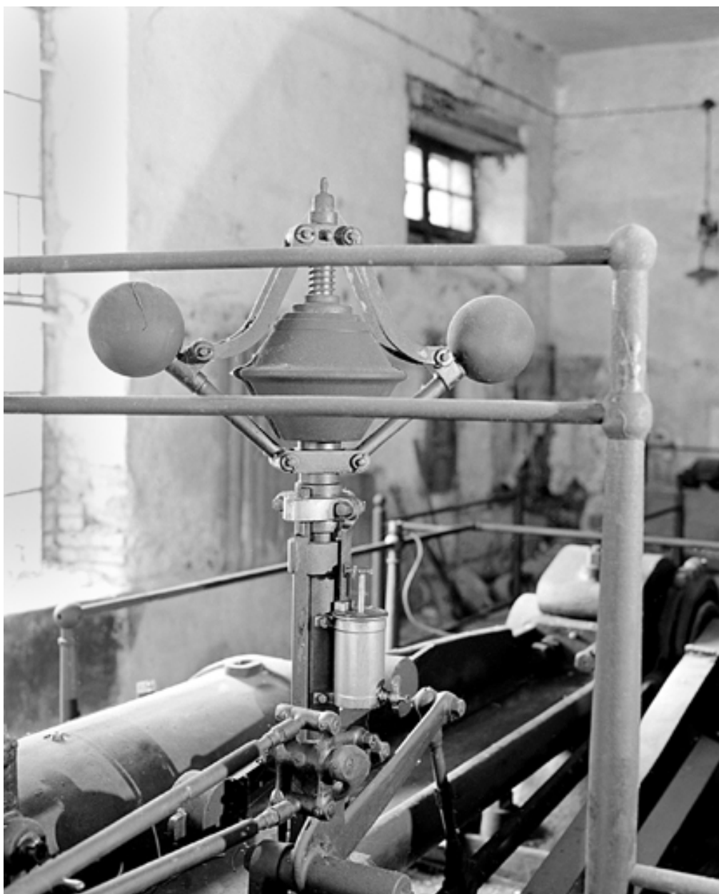
Régulateur à boules.
