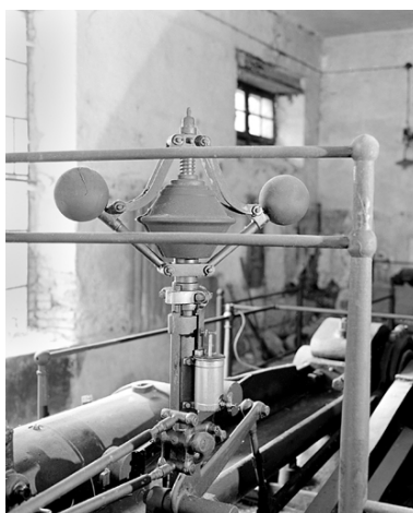
Régulateur à boules. Phot. Yves Sancey IVR43_19999000229X
