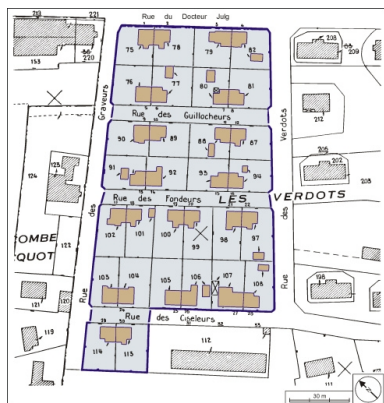
Plan-masse et de situation. Extrait du plan cadastral, 1979, section AC, 1:1000. Dess. André Céréza IVR43_20039000006NUDA
