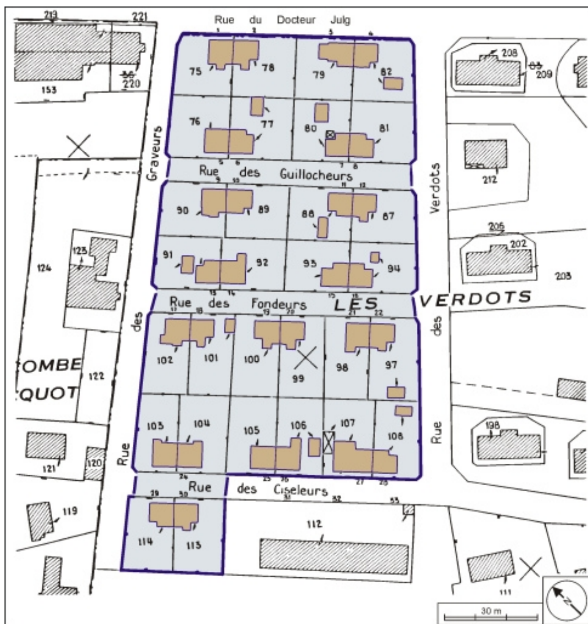
Plan-masse et de situation. Extrait du plan cadastral, 1979, section AC, 1:1000.
