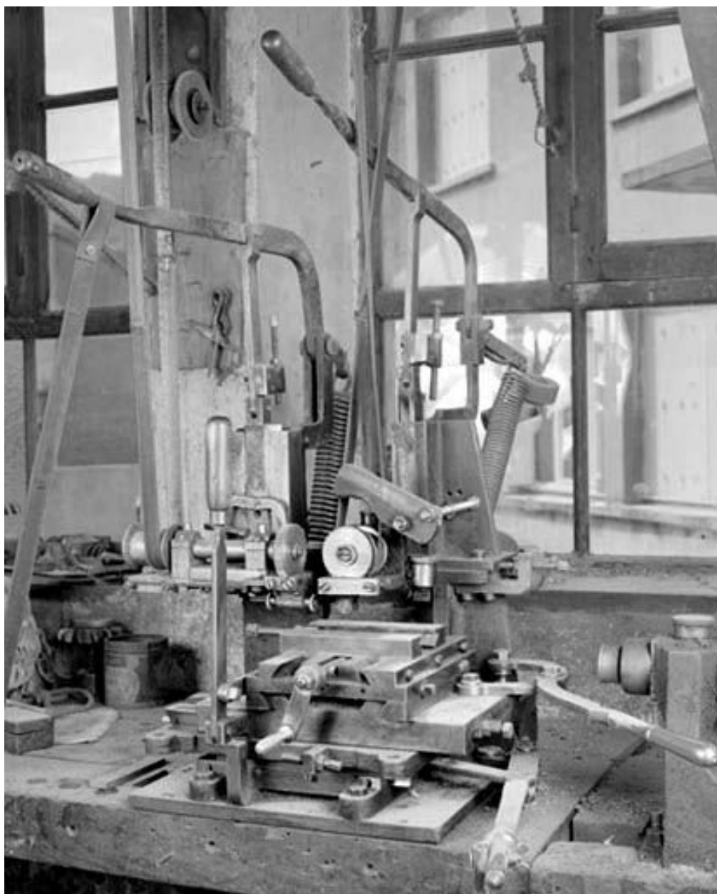
Machine à fraiser : machine à équarrir dite machine infernale.
