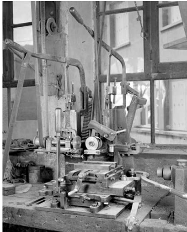
Machine à fraiser : machine à équarrir dite machine infernale. Phot. Jérôme Mongreville IVR43_19923900534X
