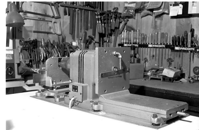
Machine à fraiser (fraiseuse- rainureuse) dite machine à chanfreiner et à faire les emplacements de charnière. Phot. Jérôme Mongreville IVR43_20003901118X
