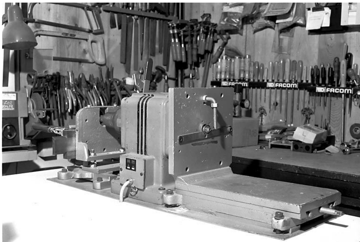
Machine à fraiser (fraiseuse-rainureuse) dite machine à chanfreiner et à faire les emplacements de charnière.
