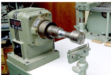
Machine à fraiser dite machine à chanfreiner le fond. Phot. Jérôme Mongreville IVR43_20003901141ZA
