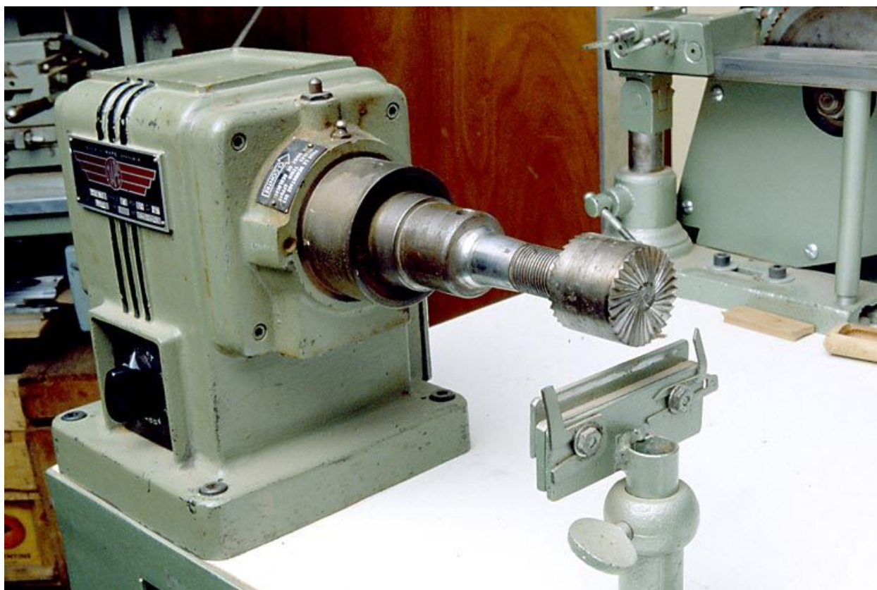
Machine à fraiser dite machine à chanfreiner le fond.
