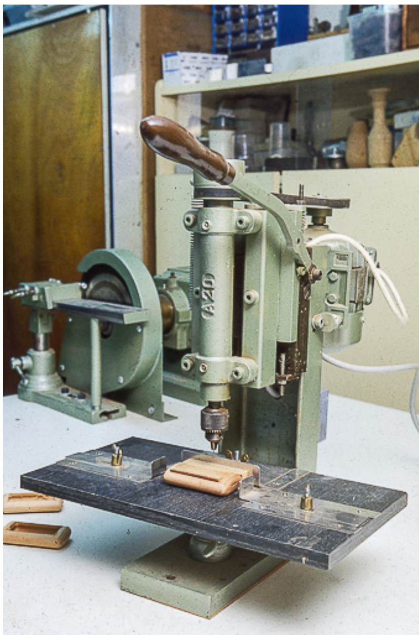
Machine à percer (perceuse sensitive).
