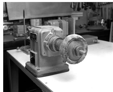
Machine à polir (tour à polir). Phot. Jérôme Mongreville IVR43_20003901116X
