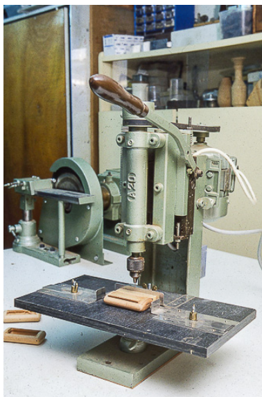
Machine à percer (perceuse sensitive). Phot. Jérôme Mongreville IVR43_20003901145ZA
