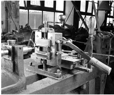
Machine à fraiser dite machine à renfoncer. Phot. Jérôme Mongreville IVR43_19923900535X
