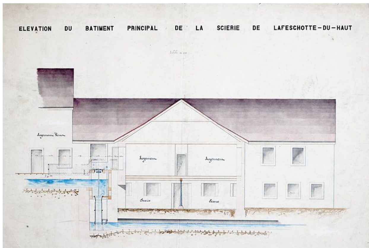
Elévation du bâtiment principal de la scierie de la Feschotte du Haut. Plan, encre, lavis, échelle 0,03/m, s.d. [fin 19e siècle].
