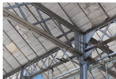
Atelier de fabrication des pompes. Détail des poutrelles de la charpente métallique. Phot. Jérôme Mongreville IVR43_20112501192NUC4A
