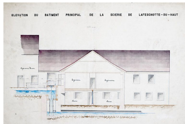
Élévation du bâtiment principal de la scierie de la Feschotte du Haut. Plan, encre, lavis, échelle 0,03/m, s.d. [fin 19e siècle]. Phot. Jérôme Mongreville, Autr. IVR43_20122501213NUC4A
