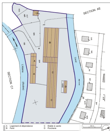
Plan-masse et de situation. Extrait du plan cadastral, 1984, section AD, 1:1000. Dess. André Céréza IVR43_20039000040NUDA
