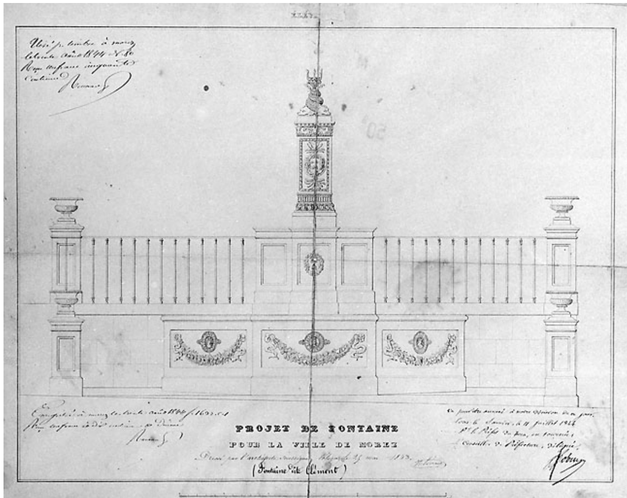
Projet de fontaine pour la ville de Morez (Fontaine dite Clément). Elévation, 1843.
