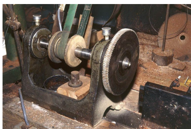
Vue d'ensemble de la machine équipée d'une fraise, de trois quarts. Phot. Jérôme Mongreville IVR43_20003901004ZA
