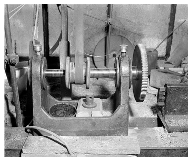
Vue d'ensemble de la machine équipée d'une fraise. Phot. Jérôme Mongreville IVR43_20003901005X
