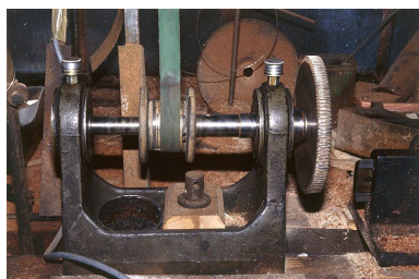
Vue d'ensemble de la machine équipée d'une fraise. Phot. Jérôme Mongreville IVR43_20003901006ZA
