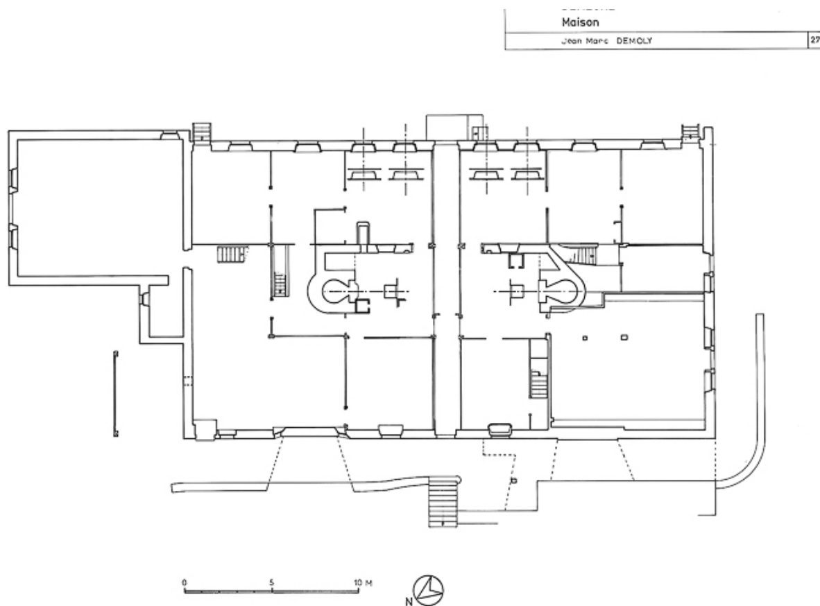
Plan au sol.
