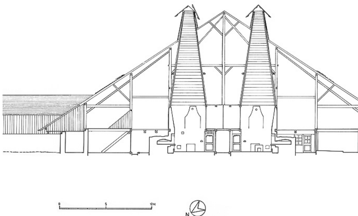
Coupe transversale.
