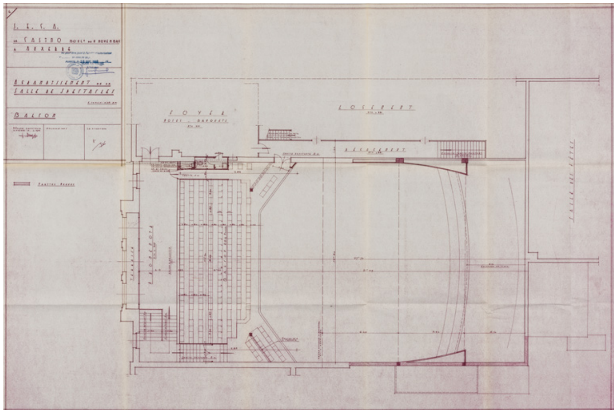
SECA Le Casino. Bould du 11 Novembre à Auxerre. Agrandissement de la salle de spectacles. Balcon. Avril 1966.
