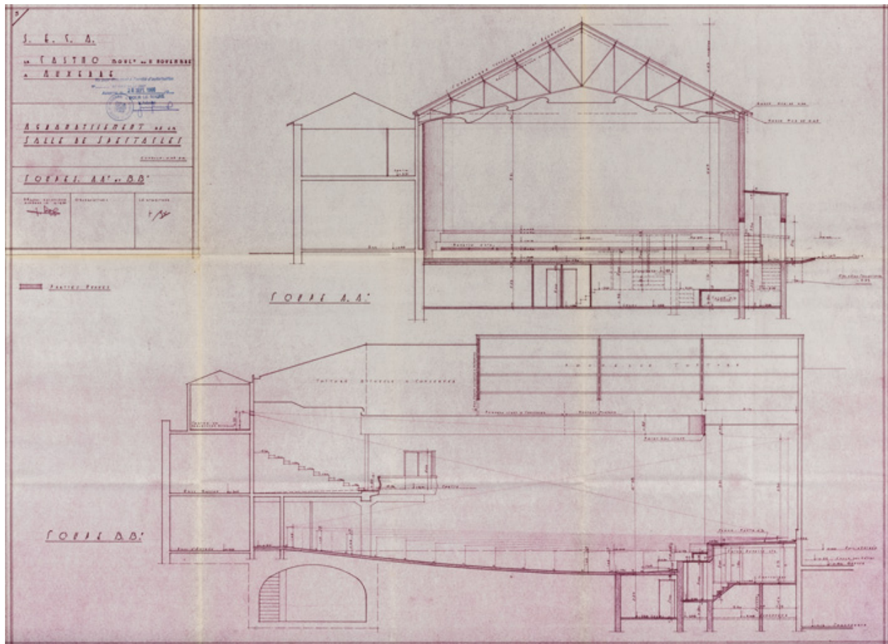
SECA Le Casino. Bould du 11 Novembre à Auxerre. Agrandissement de la salle de spectacles. Coupes AA' et BB'. Avril 1966.
