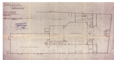
Grand Casino Auxerrois. Rez de chaussée. Etat des lieux. S.d. [1959]. Phot. Pierre-Marie Barbe- Richaud, Autr. Pierre Mégiès IVR26_20238900827NUC2A
