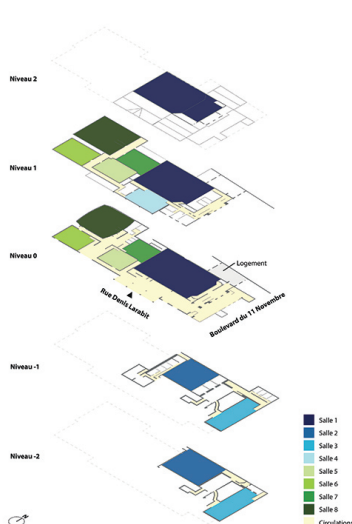
Croquis de répartition des salles par niveau (d'après des plans non signés fournis par la direction).
