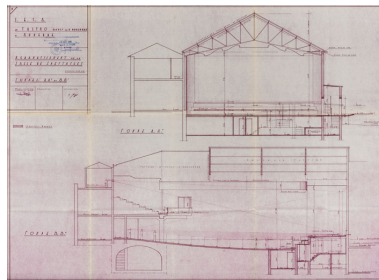
SECA Le Casino. Bould du 11 Novembre à Auxerre. Agrandissement de la salle de spectacles. Coupes AA' et BB'. Avril 1966. Phot. Pierre-Marie Barbe- Richaud, Autr. Pierre Mégiès IVR26_20238900826NUC4A
