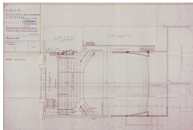
SECA Le Casino. Bould du 11 Novembre à Auxerre. Agrandissement de la salle de spectacles. Balcon. Avril 1966. Phot. Pierre-Marie Barbe- Richaud, Autr. Pierre Mégiès IVR26_20238900825NUC4A
