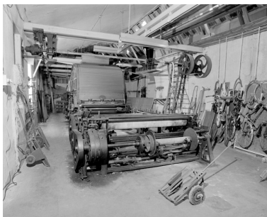
Encolleuse de la Société Alsacienne de Constructions Mécaniques. Phot. Yves Sancey IVR43_19999000244X
