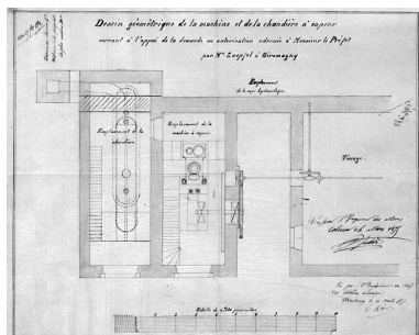
Dessin géométrique de la machine et de la chaudière à vapeur servant à l'appui de la demande
