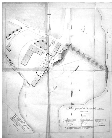
Usine de la Saisse. Plan général [...]. Phot. Jérôme Mongreville IVR43_19963900212X
