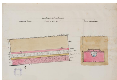
Coupes sur une canalisation (1895). Phot. Pierre-Marie Barbe- Richaud, Autr. Frédéric Delafond, Autr. François Dulac IVR26_20217100335NUC4A
