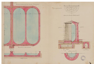
Plan des bassins de refroidissement, plan et coupe du château d'eau (1895). Phot. Pierre-Marie Barbe- Richaud, Autr. Frédéric Delafond, Autr. François Dulac IVR26_20217100334NUC4A
