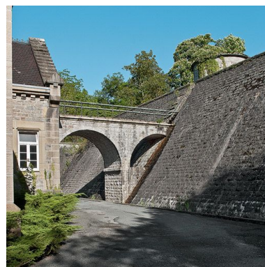
Aqueduc entre le réservoir et les bains d'Aligre (à gauche). Phot. Pierre-Marie Barbe-Richaud IVR26_20107100983NUC2AQ
