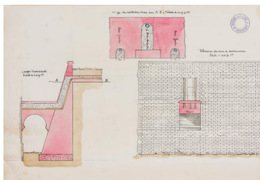
Mur de soutènement derrière les bains d'Aligre (1895). Phot. Pierre-Marie Barbe- Richaud, Autr. Frédéric Delafond, Autr. François Dulac IVR26_20217100333NUC4A
