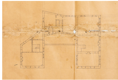
Plan du rez-de-chaussée. Phot. Pierre-Marie Barbe- Richaud, Autr. auteur inconnu IVR26_20205800332NUC4A
