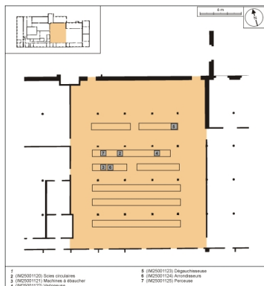
Plan de localisation des machines de la ligne de fabrication des têtes de pipe en bruyère. Atelier principal.
