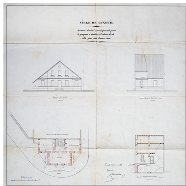
Plan, coupe et élévations. Phot. Jérôme Mongreville, Autr. Félix-Hercule Grandmougin IVR43_20207000440NUC4A
