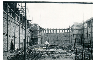
Chantier de l'église Saint-Joseph de Besançon : vue de la nef en construction s.d. [1952-1953]. Autr. René Tournier IVR43_20212500155NUC4A
