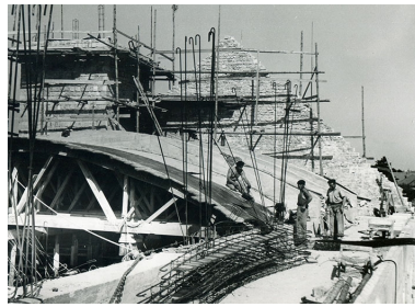
Chantier de l'église Saint-Joseph de Besançon : vue du coffrage en bois de la voûte. s.d. [1953]. Autr. René Tournier IVR43_20212500154NUC4A
