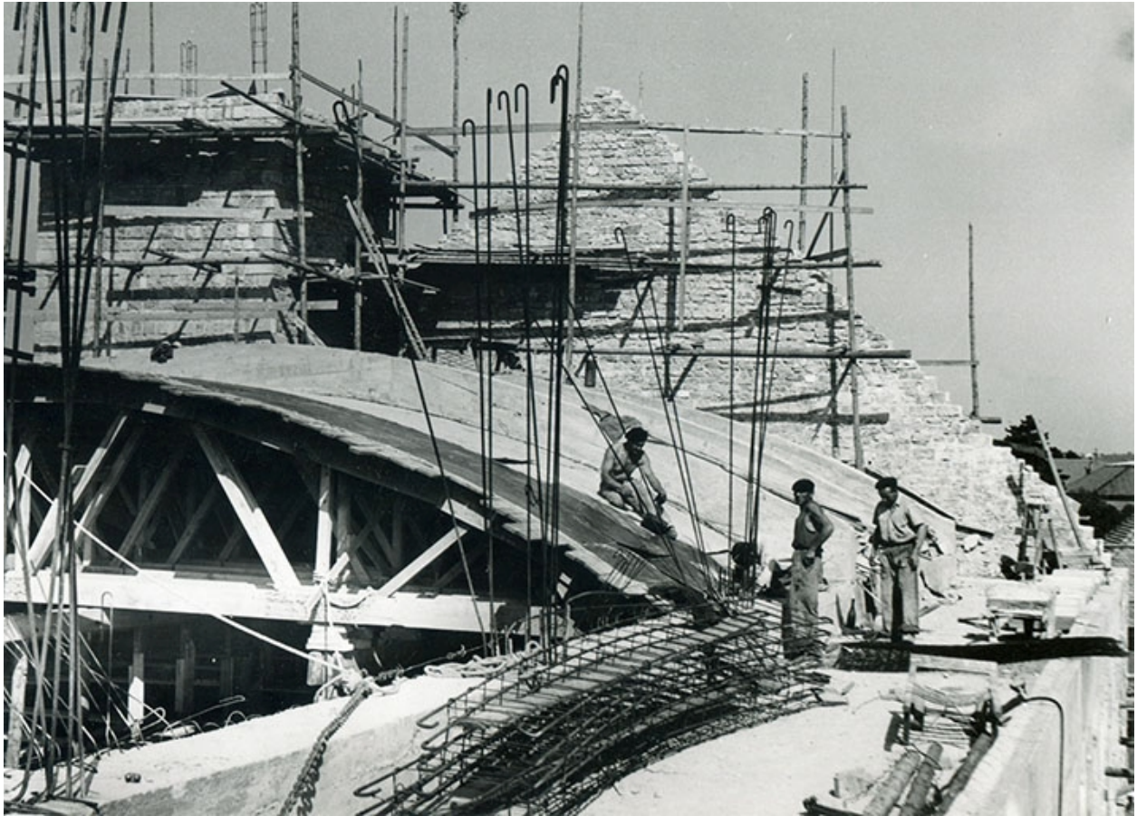
Chantier de l'église Saint-Joseph de Besançon : vue du coffrage en bois de la voûte. s.d. [1953].
