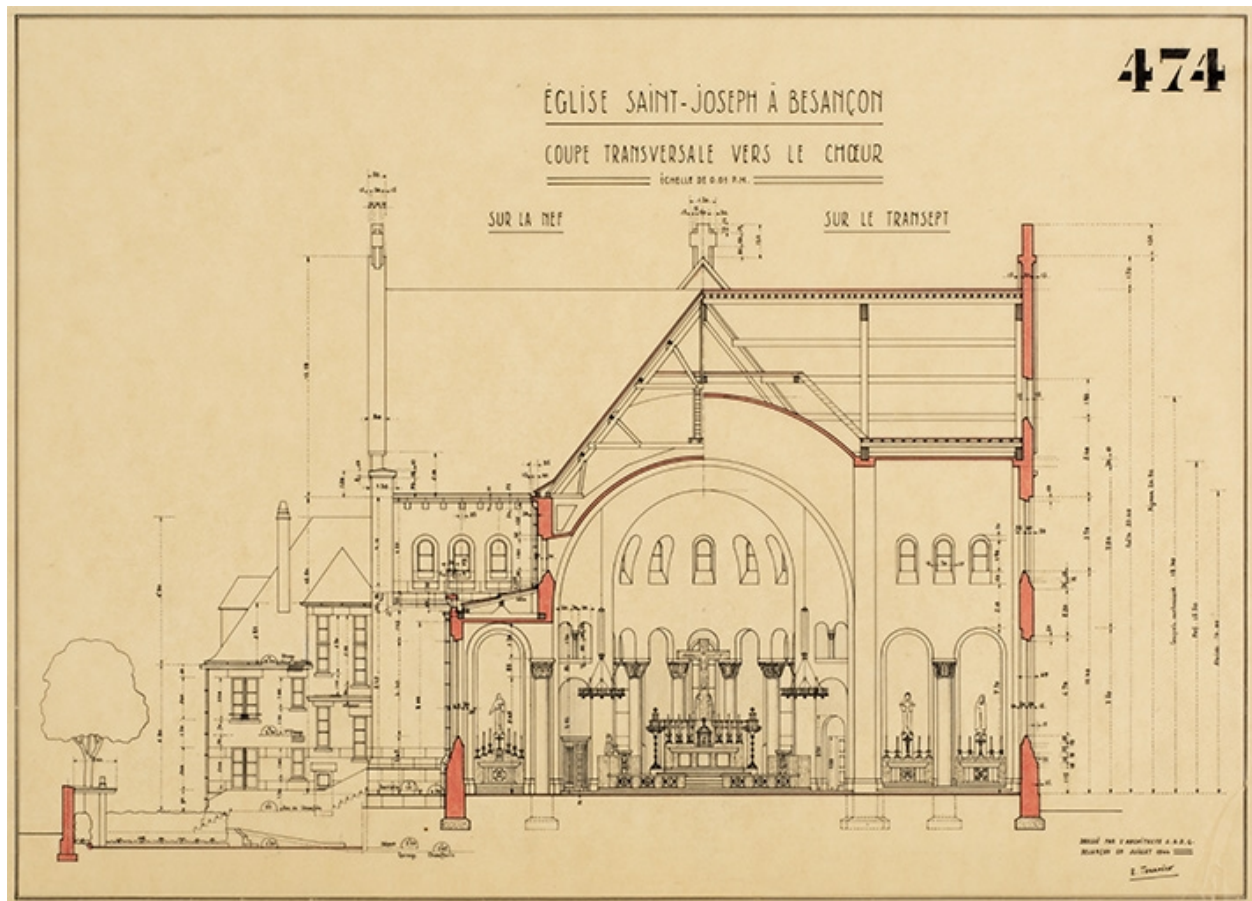
Église Saint-Joseph à Besançon. Coupe transversale vers le chœur [projet non réalisé]. Juillet 1944.
