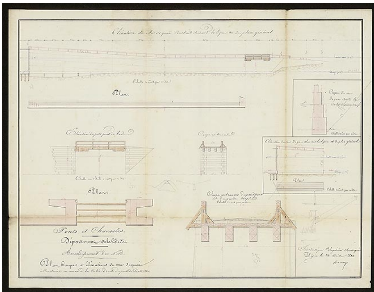
Elévation du mur de quai construit suivant la ligne ac du plan général. 1832.
