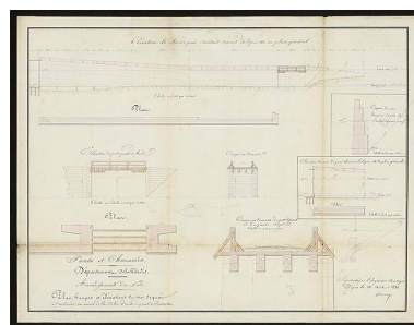
Elévation du mur de quai construit suivant la ligne ac du plan général. 1832. Phot. Petot Frédéric IVR26_20202100114NUC4A
