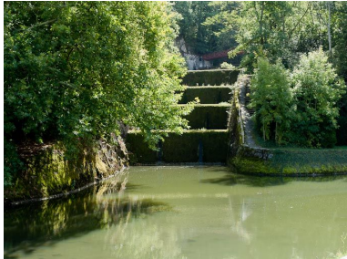
Vue des différents tabliers du déversoir.
