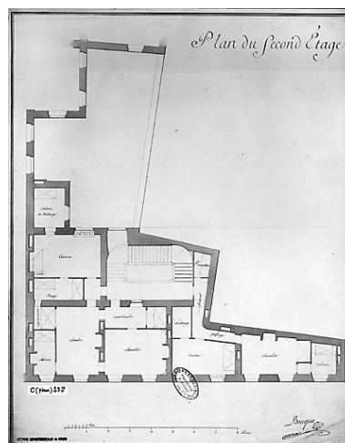
Plan du second étage.
