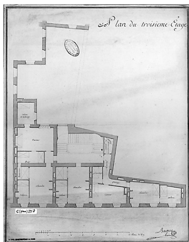
Plan du troisième étage.
