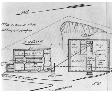
Société fromagère des Mouilles. Bellecombe. Construction d'un chalet de fromagerie avec porcherie [détail : plan des bâtiments]. Phot. Jérôme Mongreville, Phot. Marcel David IVR43_19943901403X
