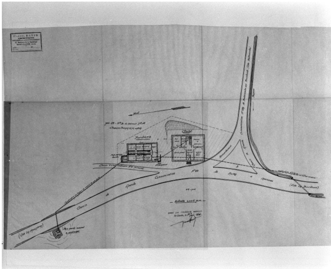
Société fromagère des Mouilles. Bellecombe. Construction d'un chalet de fromagerie avec porcherie. Plan général de l'installation.
