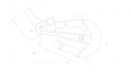
Boulevard des Filles. Plan du niveau 1. Dess. Alain Morelière IVR26_20122100045A0YY
