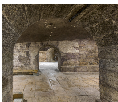
Caves, rez-de-chaussée : passages pour accéder aux différents vaisseaux. Phot. Pierre-Marie Barbe-Richaud IVR26_20152100894NUC4A
