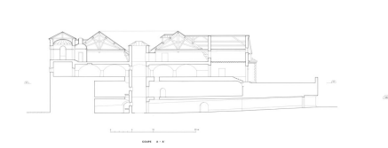
Boulevard des Filles. Coupe A-A'. Dess. Alain Morelière IVR26_20122100048A0YY
