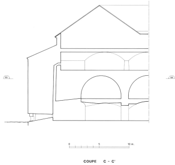
Boulevard des Filles. Coupe C-C'. Dess. Alain Morelière IVR26_20122100050A0YY
