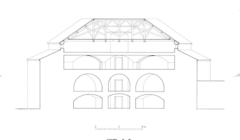
Boulevard des Filles. Coupe B-B'. Dess. Alain Morelière IVR26_20122100049A0YY
