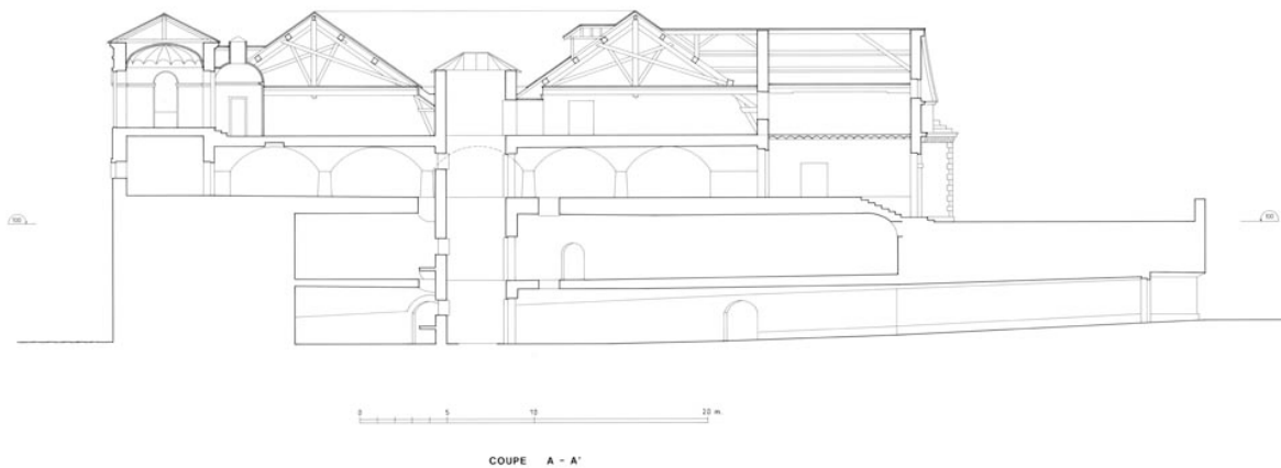
Boulevard des Filles. Coupe A-A'.
