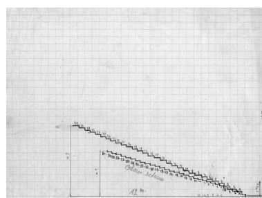
[Coupe des gradins]. S.d. [1945 ou 1946]. Autr. auteur inconnu IVR26_20242100227NUC4A
