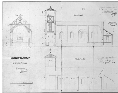
Coupe en travers, coupe en longueur, élévation latérale. Phot. Yves Sancey, Autr. René Léon Victor Pourchot IVR43_19833900765V
