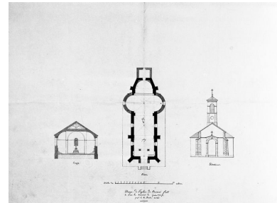
Coupe, plan et élévation. Phot. Yves Sancey, Autr. Claude-Guillaume (entrepreneur) Boin IVR43_19833900764V
