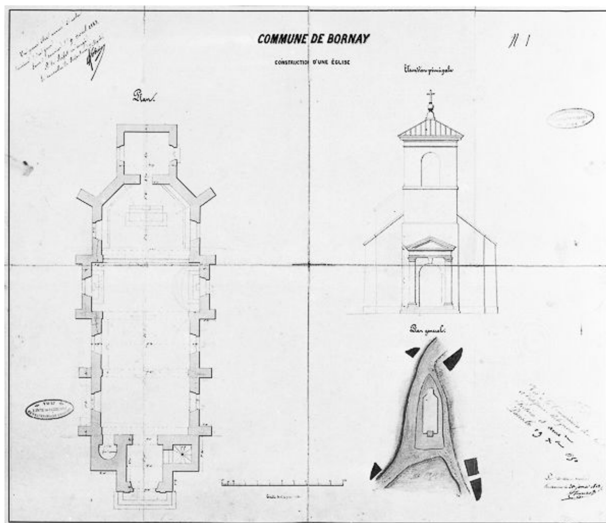
Plan, élévation principale, plan général.
