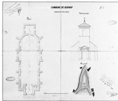
Plan, élévation principale, plan général. Phot. Yves Sancey, Autr. René Léon Victor Pourchot IVR43_19833900766V
