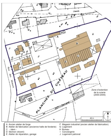
Plan-masse et de situation. Extrait du plan cadastral numérisé, 2008, section AM, échelle 1:1000 réduit à 1:1250. Source : Direction générale des Finances Publiques - Cadastre ; mise à jour : 2008. Dess. André Céréza IVR43_20087000158NUDA
