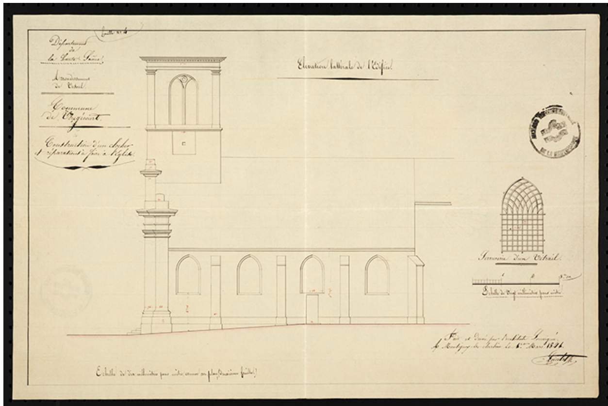
Construction d'un clocher et réparation à faire à l'église. [Elévation latérale de l'église] 1841
