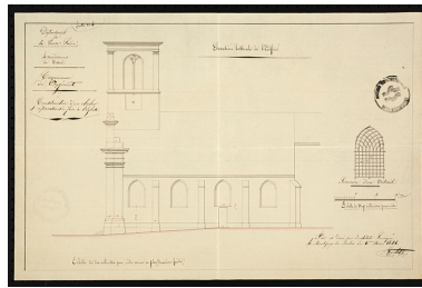
Construction d'un clocher et réparation à faire à l'église. [Elévation latérale de l'église] 1841 Phot. Sonia Dourlot IVR43_20167000120NUC4A
