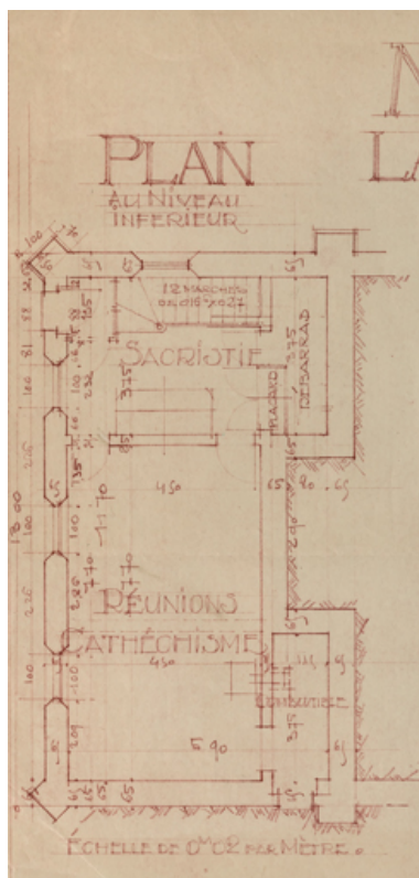
Plan du niveau inférieur de l'église : la sacristie et la salle de catéchisme, 1950. Autr. Lazare Bertrand, Phot. Pierre-Marie Barbe-Richaud IVR26_20248900113NUC4A
