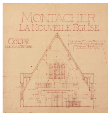
Coupe transversale : vue sur l'entrée, 1950. Autr. Lazare Bertrand, Phot. Pierre-Marie Barbe-Richaud IVR26_20248900116NUC2A
