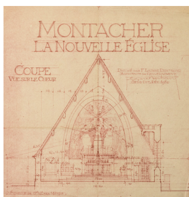
Coupe transversale : vue sur le chœur, 1950. Autr. Lazare Bertrand, Phot. Pierre-Marie Barbe-Richaud IVR26_20248900117NUC2A
