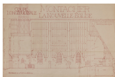
Coupe longitudinale de l'église, 1950. Autr. Lazare Bertrand, Phot. Pierre-Marie Barbe-Richaud IVR26_20248900111NUC4A
