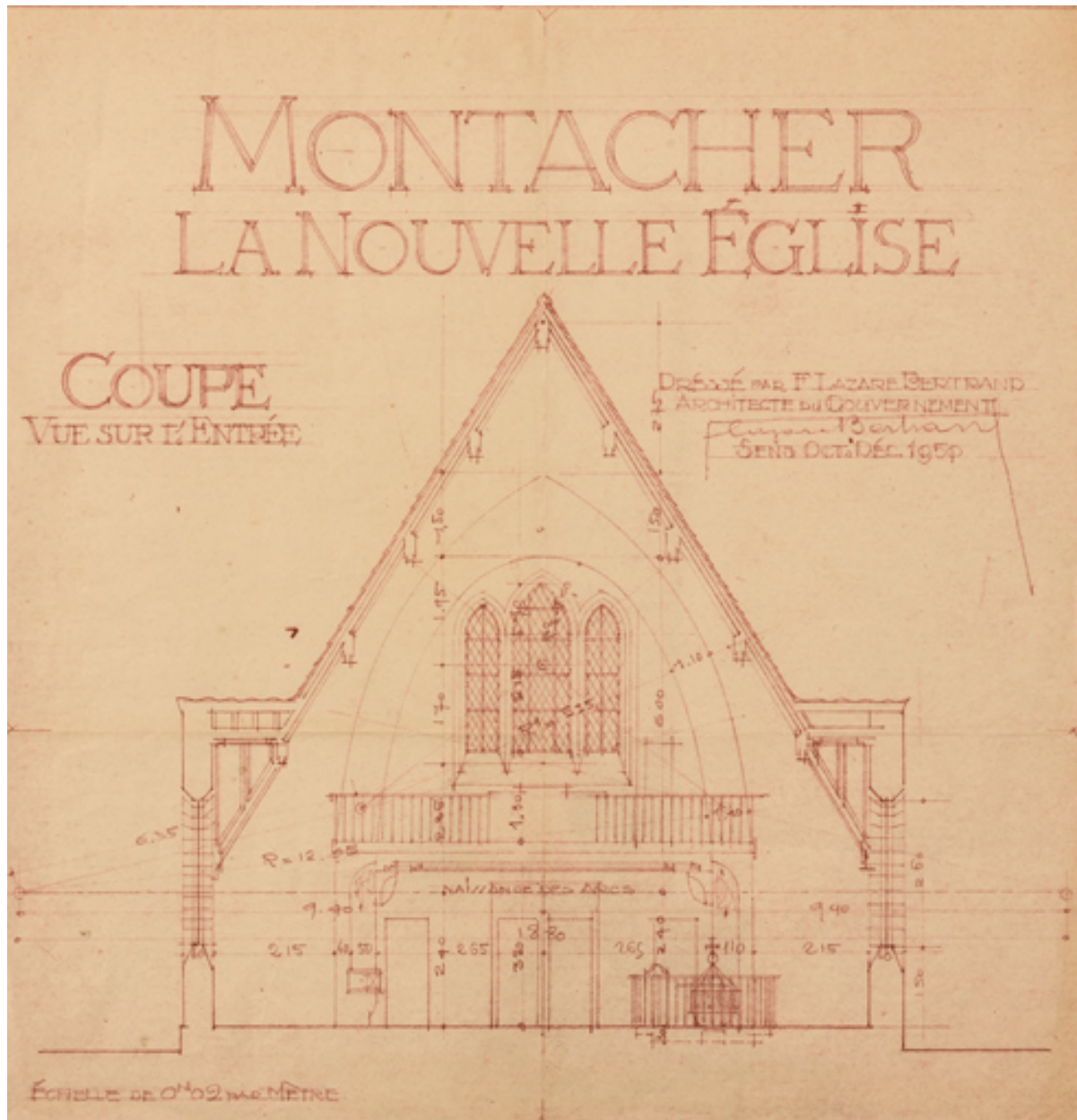
Coupe transversale : vue sur l'entrée, 1950.
