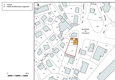
Plan-masse et de situation. Extrait du plan cadastral, 2017, section AC, 1/1 000. Dess. Bertrand Turina IVR43_20182501352NUDA
